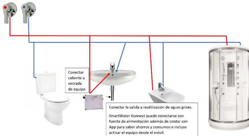
PLANO SMARTWATER KONNECT A SISTEMA DE AGUAS GRIS
