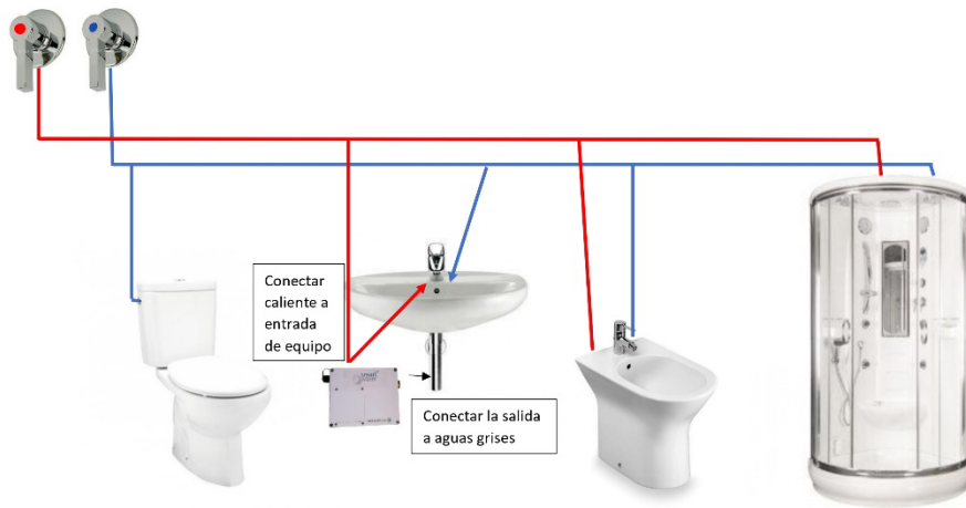
PLANO SMARTWATER HOME A SISTEMA DE AGUAS GRISES
